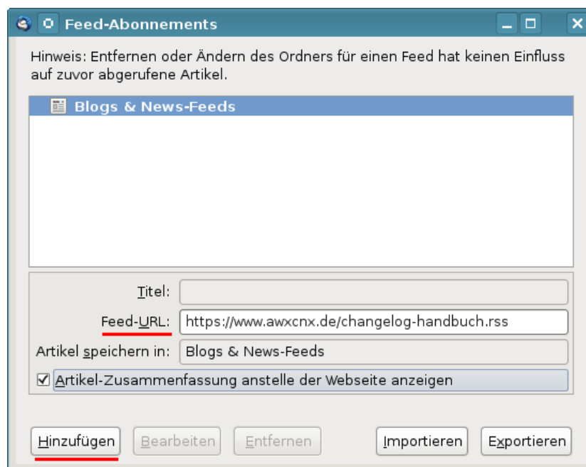
Abbildung 9.10: RSS-Feed hinzufügen
